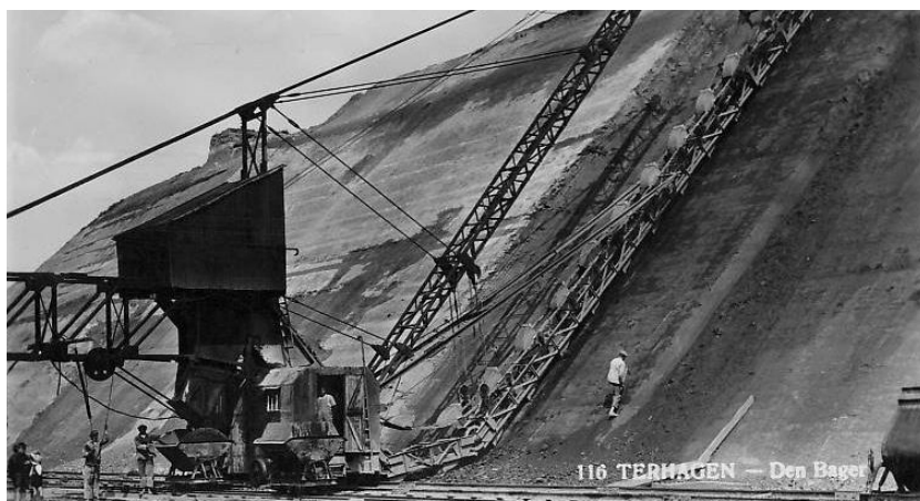
Kleibagger
